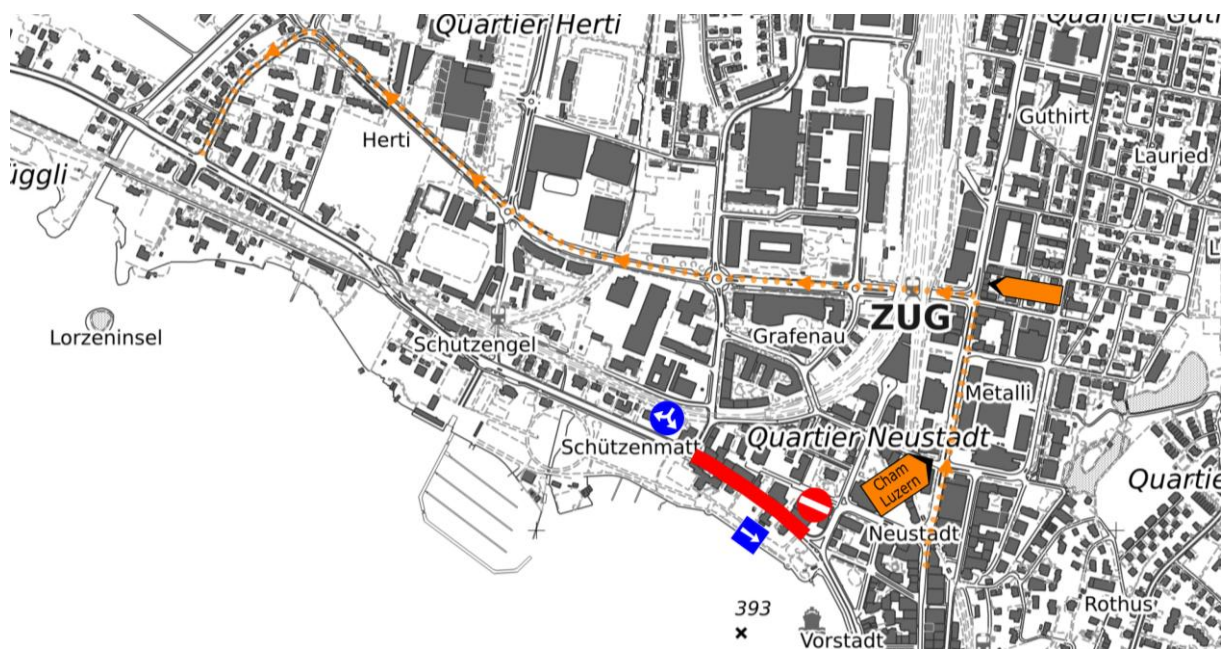
Übersichtsplan: Umleitungskonzept bei der Teilspernung
